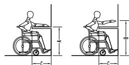
Alcance frontal sobre obstáculo (quando 0,50 < C \leq 0,60 m)
